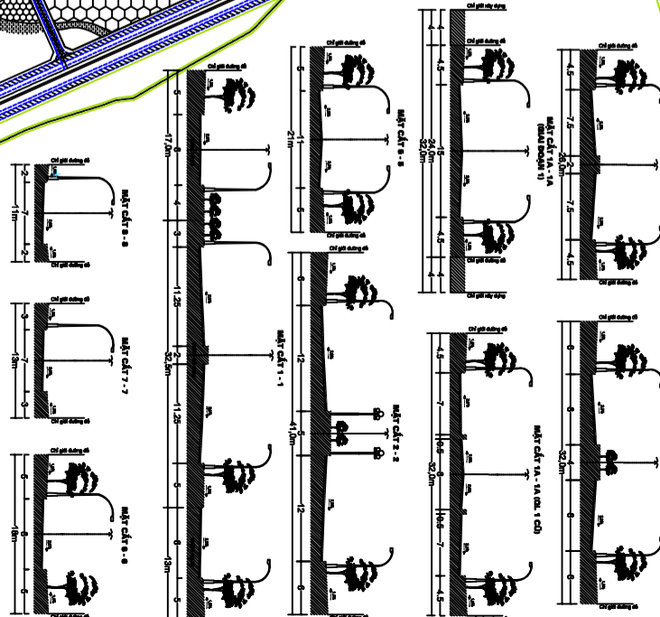
MẶT CẮT NGANG ĐƯỜNG ĐIỂN HÌNH
